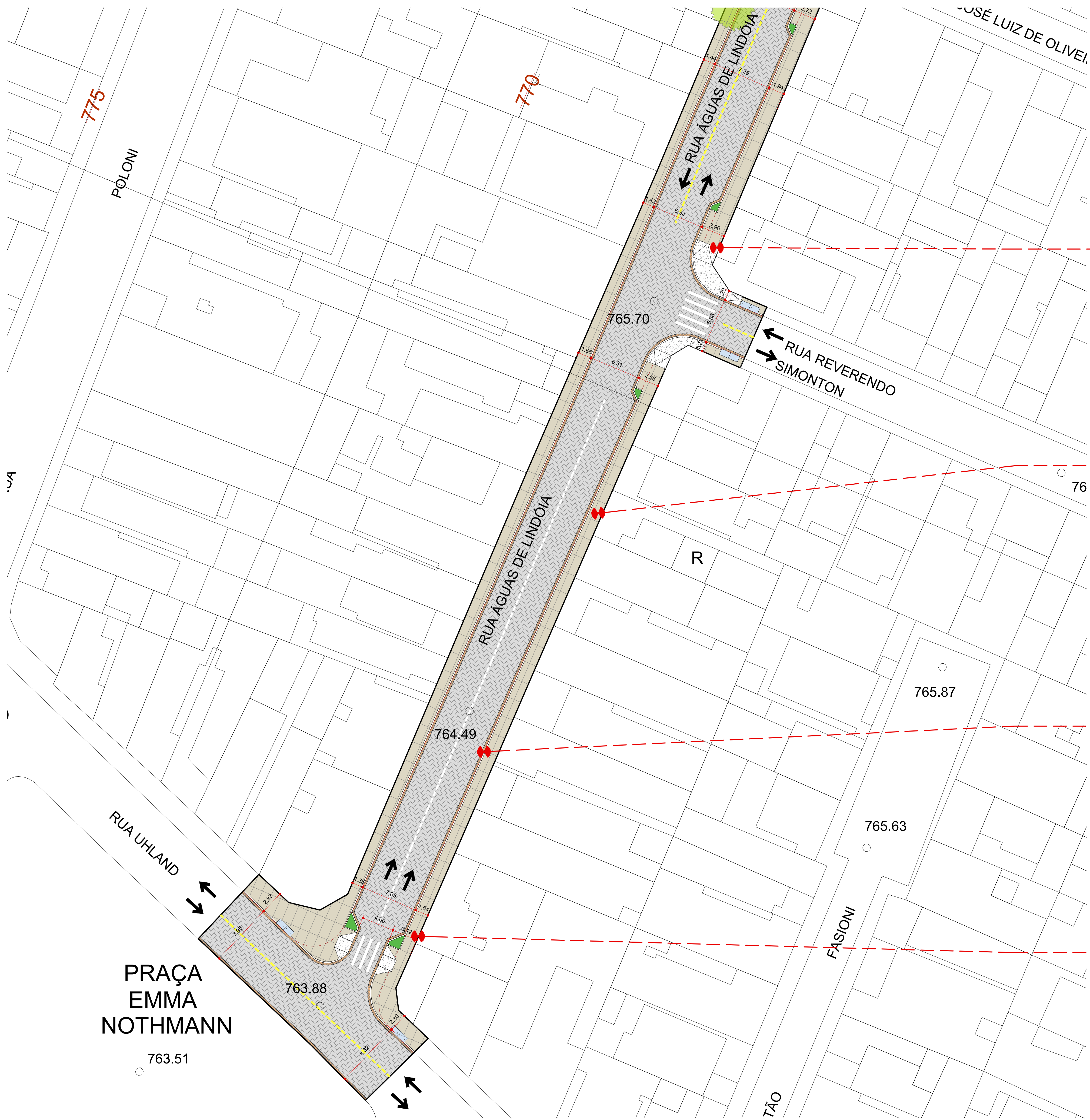
ALARGAMENTO DE ESQUINAS ADJACENTE A TRAVESSIAS
