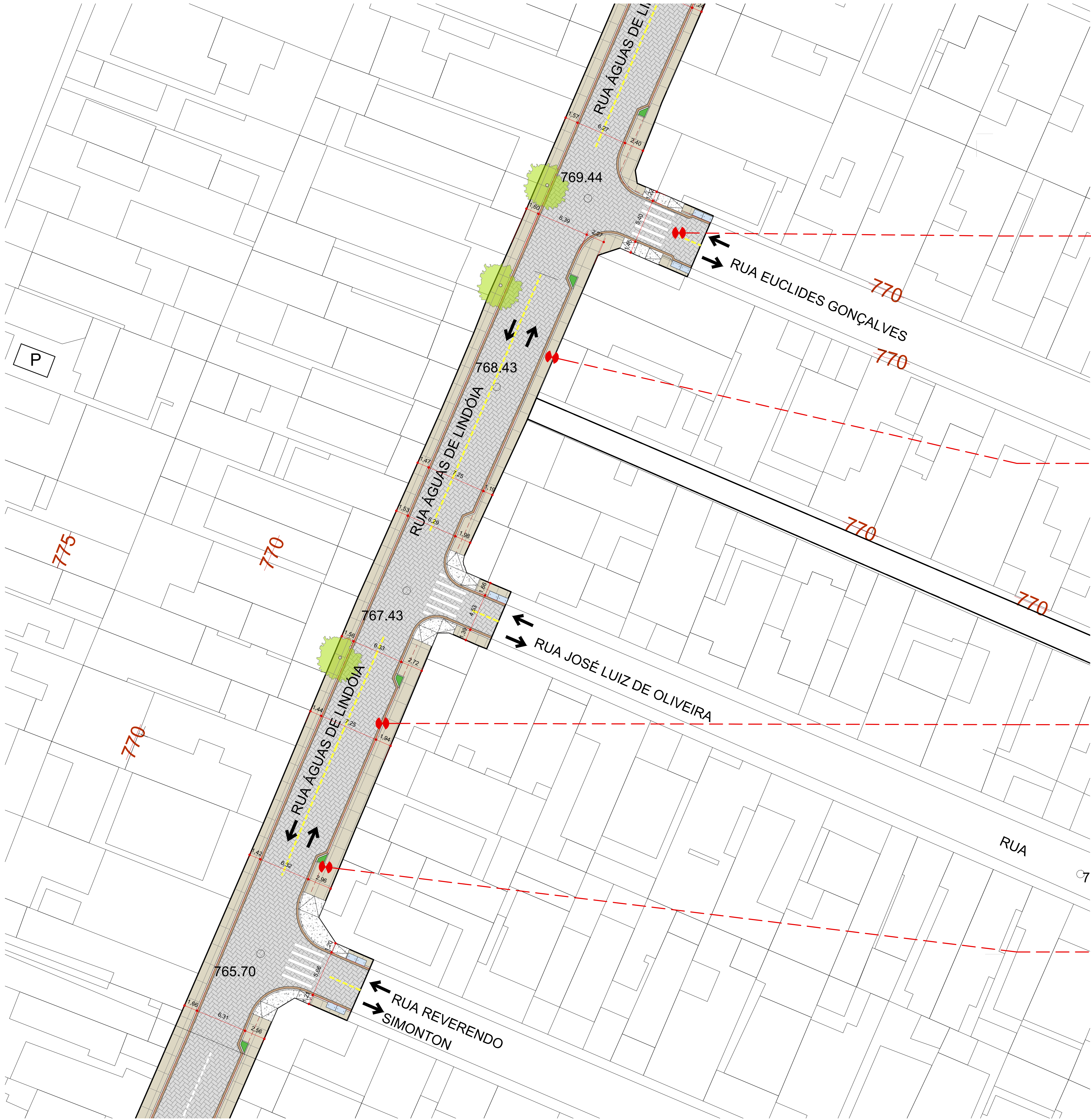
PLANTA DE URBANISMO FUNCIONAL - TRECHO 02 ESC. 1:250
